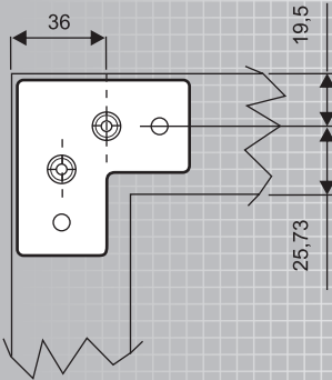
C7317 соединительный уголок для профиля E7141
