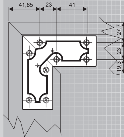
C7317 соединительный уголок для профиля E7141
