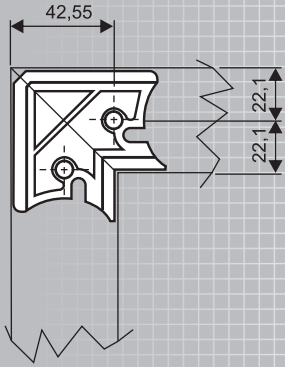
C7059 соединительный уголок для профилей B26116/E9805/H24693
